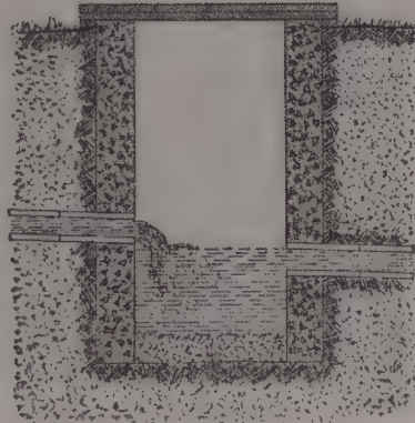
Fig. 64. A silt basin.
